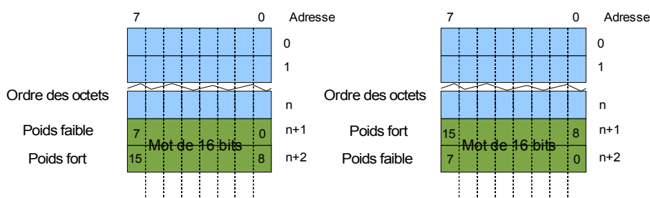
Fig. 9. Différents ordres d'octet
