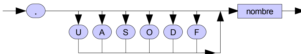
Fig. 5. Syntaxe des indicateurs de données
